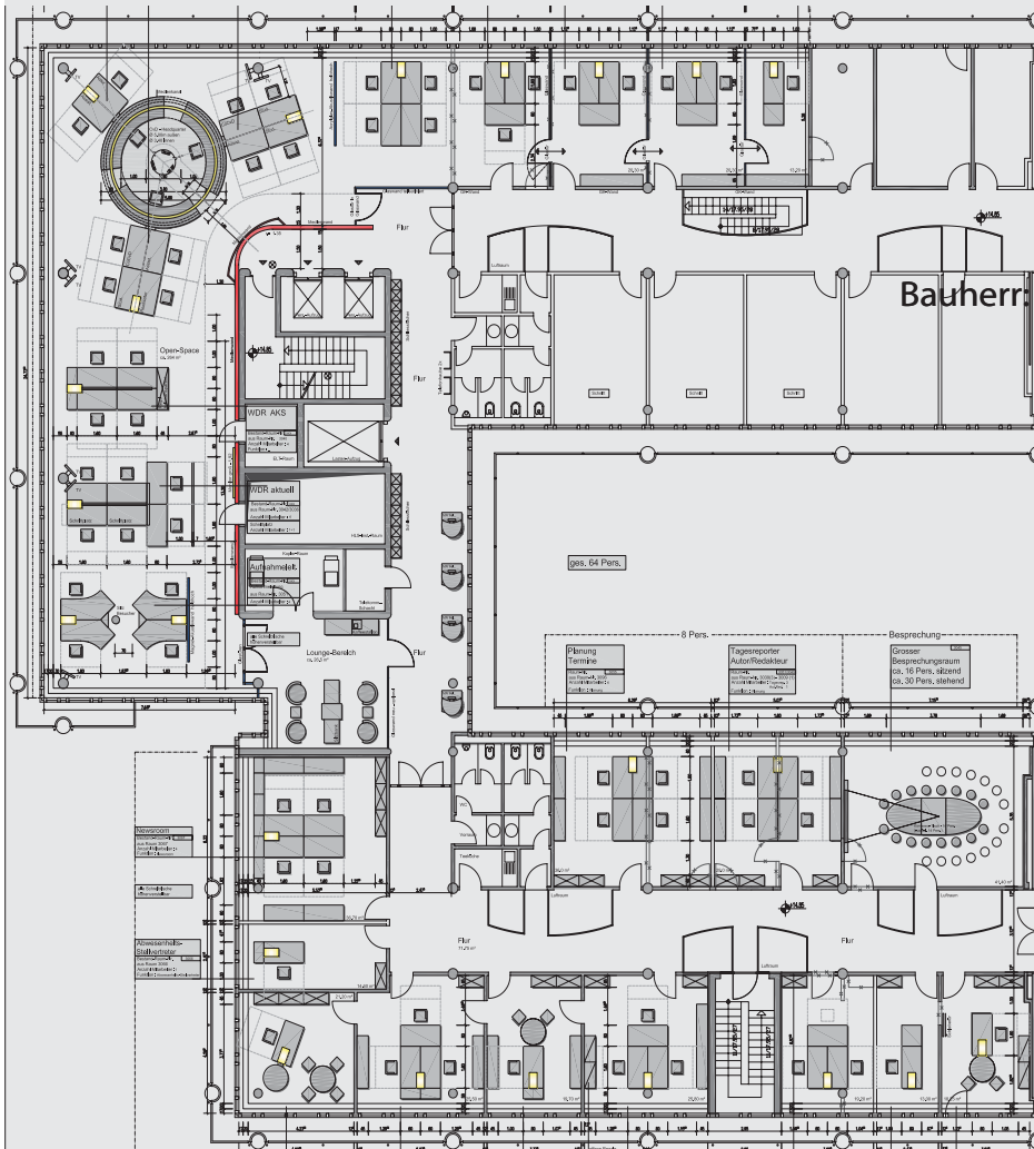
Entwurfskonzept - 3. Obergeschoss - WDR Düsseldorf
